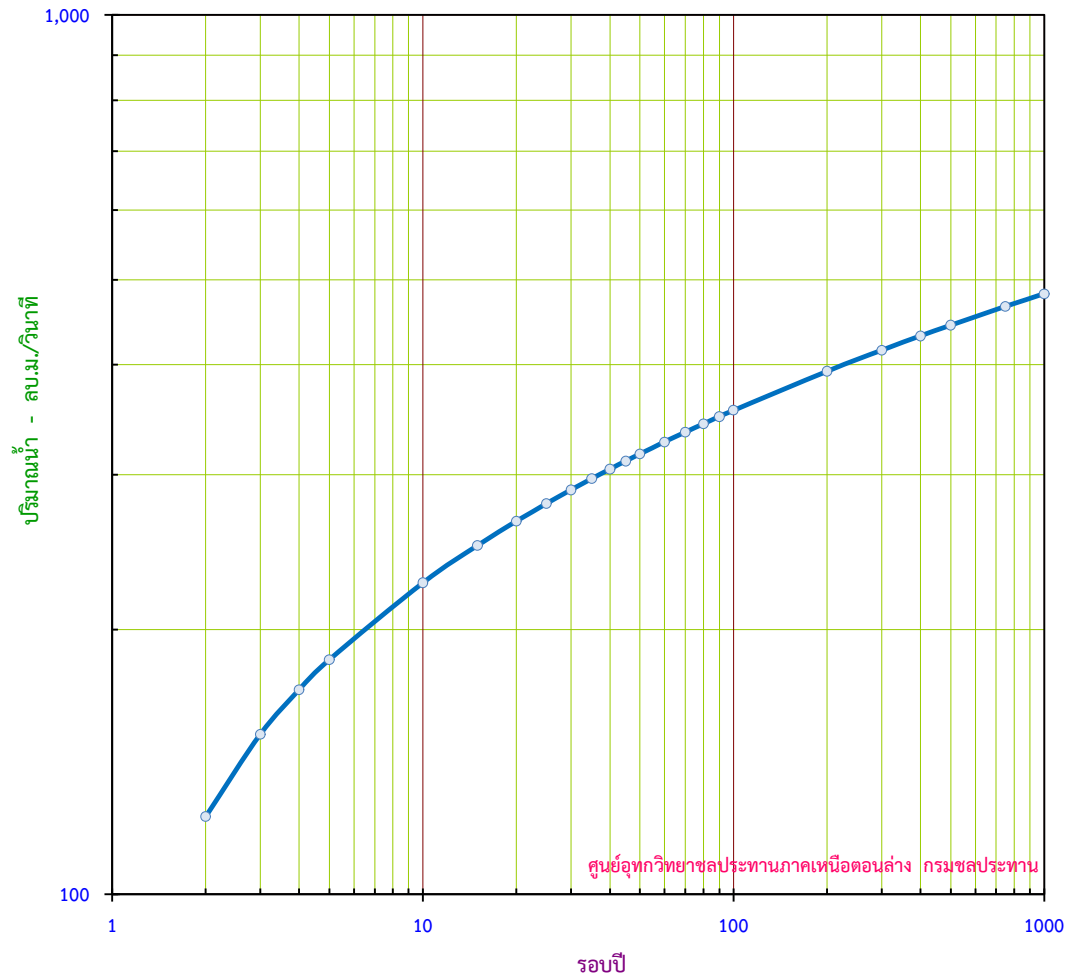
กราฟแสดง ปริมาณน้ำสูงสุดรายปี ขนาดรอบปีต่างๆ สถานี N.55 บ.ท่าสะแก อ.ชาติตระการ จ.พิษณุโลก
